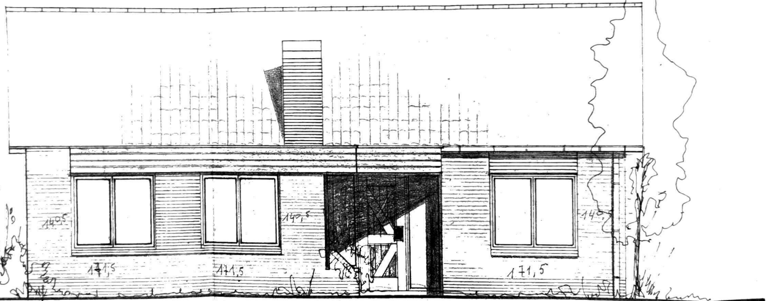
VOORGEVEL
