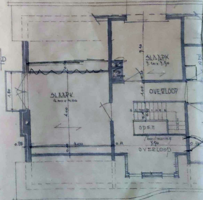
VERDIEPING
