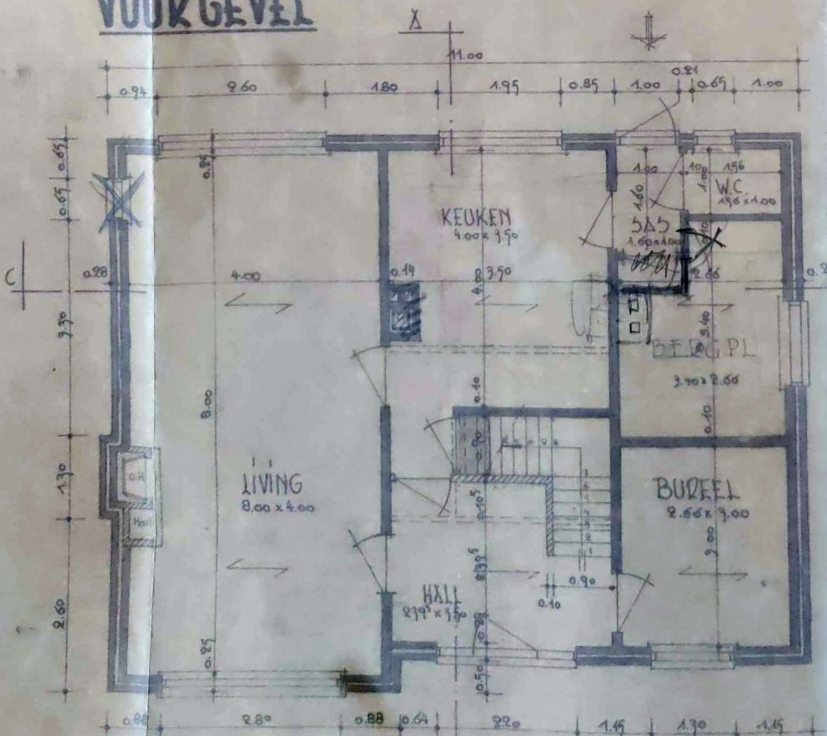
GELIJKVLOERS
