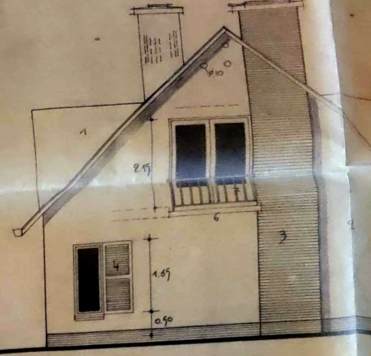
LINVERGEVEL
